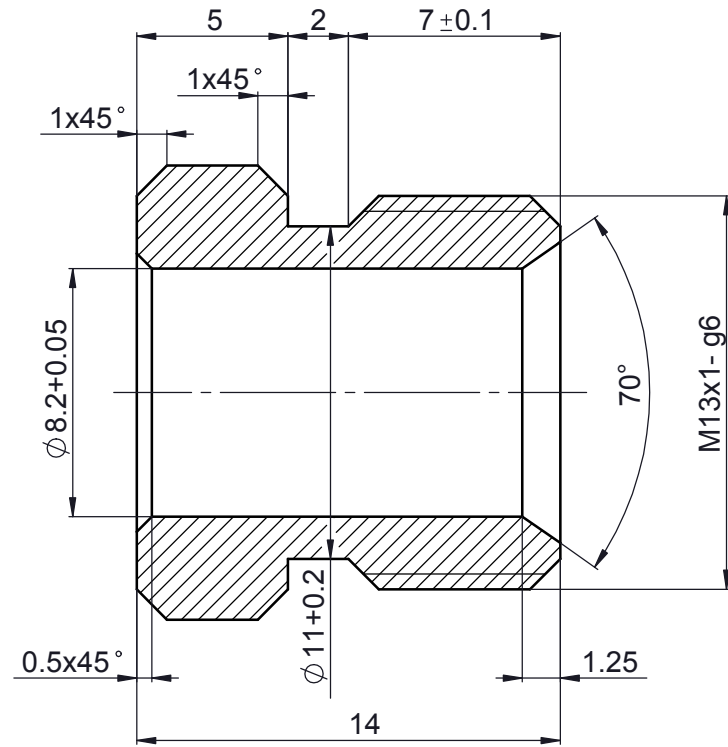
A-A (4 : 1)
